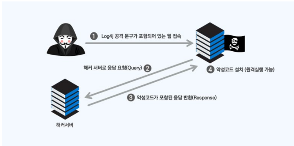
Log4j의 웹서버 공격 유형
